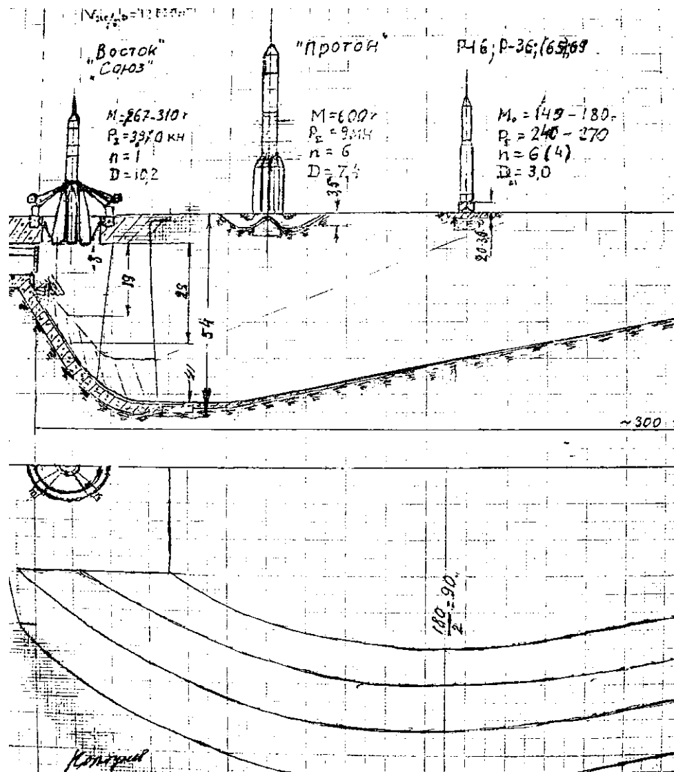
Фото 5. К уменьшению размеров и стоимости пусковых установок для ракет по предложениям автора.
